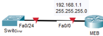
Görsel 3.18: Ethernet arayüz yapılandırma
