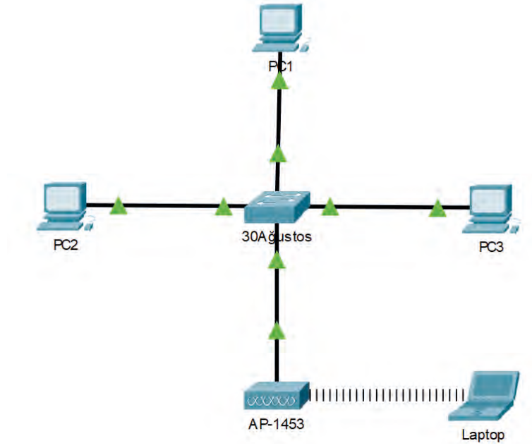
Görsel 2.53: Kablosuz ağ simülasyonu
