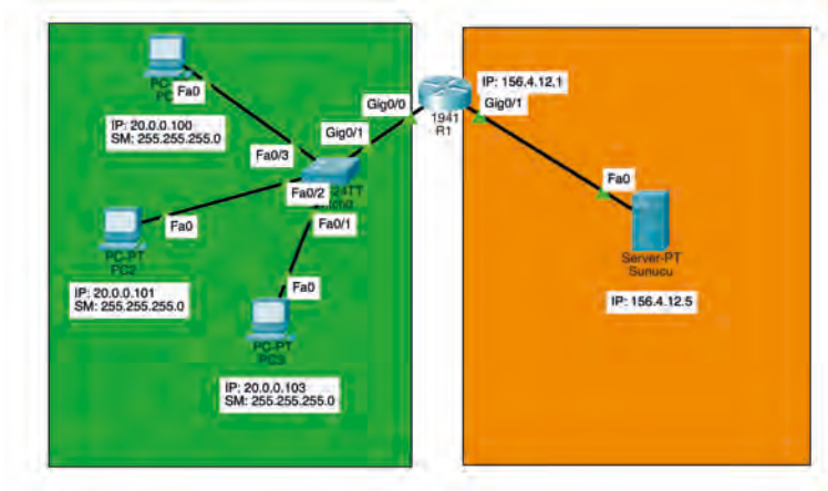
Görsel 4.24: Ağ topolojisi
