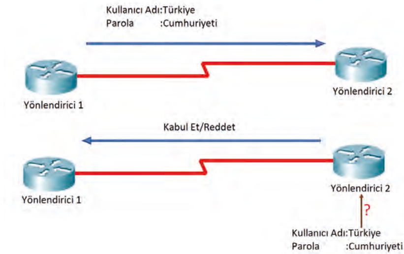
Görsel 6.2: PAP ile kimlik doğrulama
