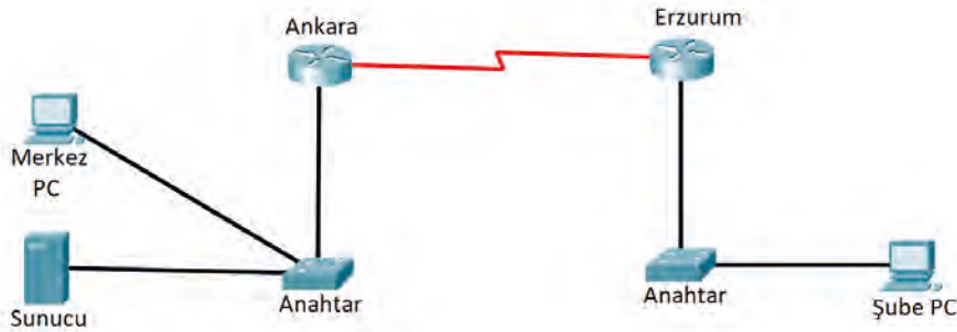
Görsel 6.4: PAP ile kimlik doğrulama ağ topolojisi
