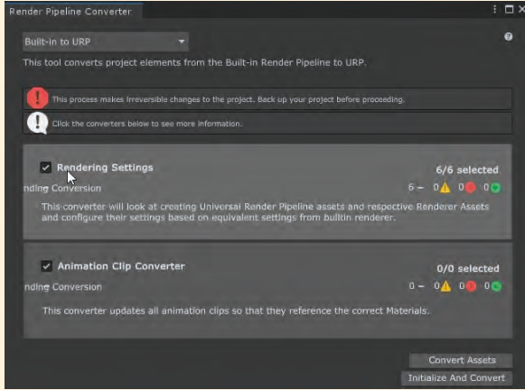
Görsel 3.42: Convert Assets ile materyal dönüşümü sağlanır.
