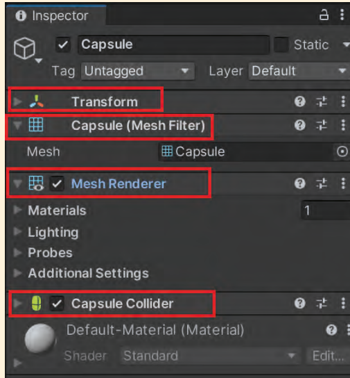
Görsel 1.10: Capsule nesnesinin bileşenleri
