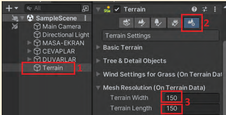
Görsel 1.58: Terrain'in boyutlarının değiştirilmesi
