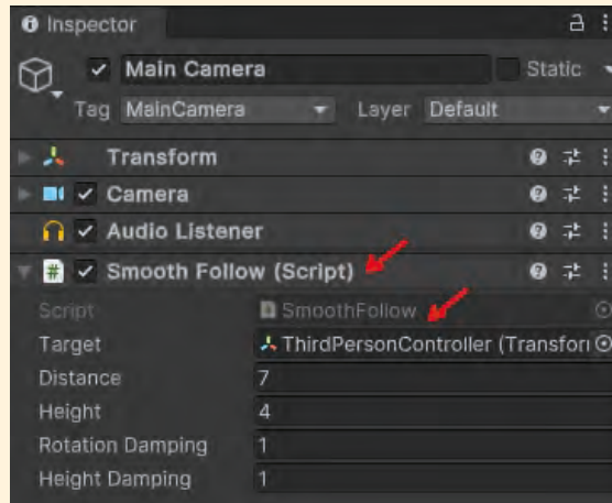
Görsel 3.145: Ana kameraya SmoothFollow kodunun eklenmesi
