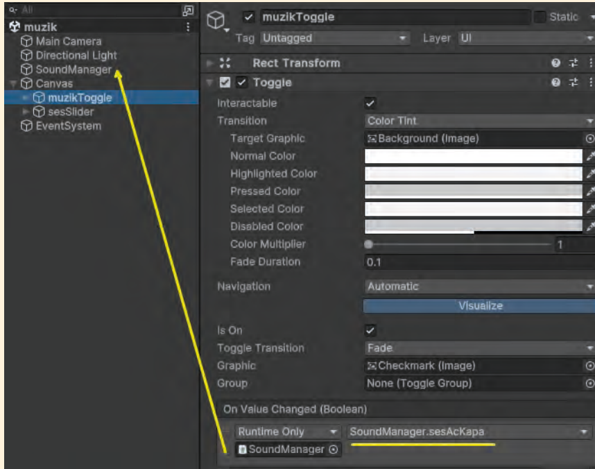
Görsel 3.154: Olayların eklenmesi
