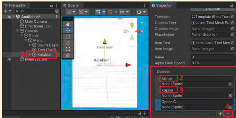
Görsel 1.100: Dropdown seçeneklerinin ayarlanması
