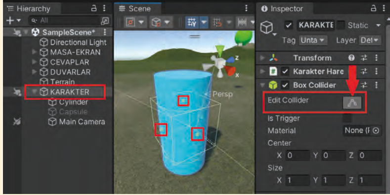
Görsel 1.85: Edit Collider düğmesi ve tutamaçlar
