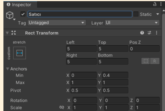
Görsel 4.22: Satıcının Rect Transform Ayarı
