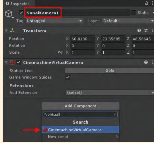
Görsel 3.6: CinemachineVirtualCamera bileşeninin eklenmesi
