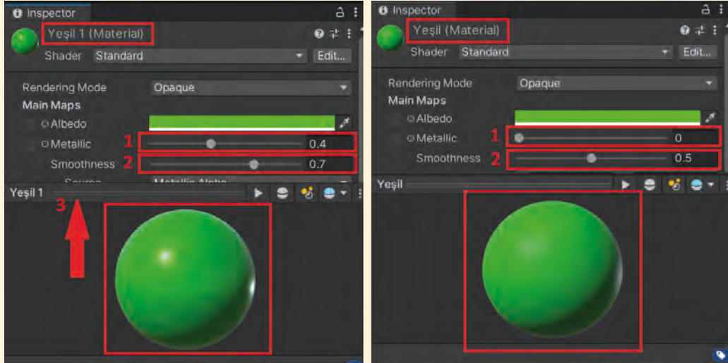
Görsel 1.45: Özellikleri farklı materyaller
