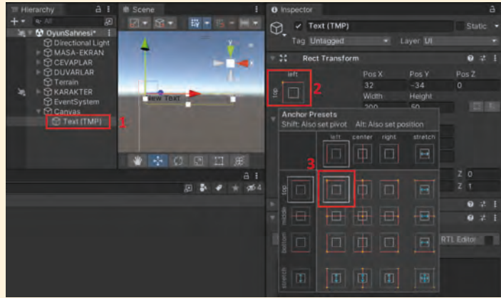
Görsel 1.112: Metin kutusunun eklenmesi ve özelliklerinin ayarlanması
