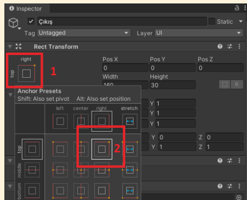
Görsel 4.12: Çıkış butonunun Rect Transform özelliğini ayarlama
