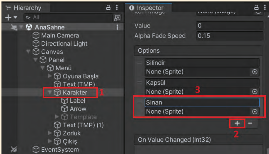
Görsel 2.78: Hazır karakter modelini oyunun karakter seçeneklerinin içerisine ekleme
