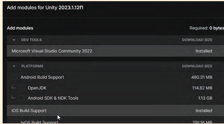
Görsel 3.124: Oyun motoruna derleme desteğinin eklenmesi
