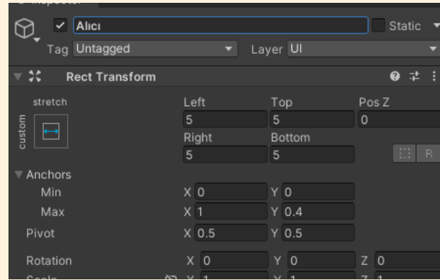
Görsel 4.23: Alıcının Rect Transform ayarı
