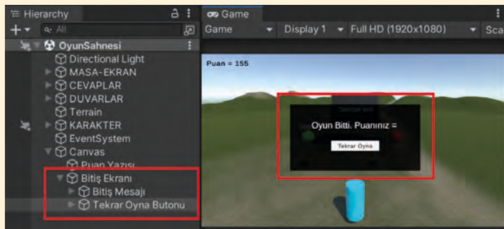
Görsel 1.114: Bitiş Ekranı'nın oluşturulması
