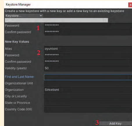
Görsel 4.76: Keystore Manager ayarları
