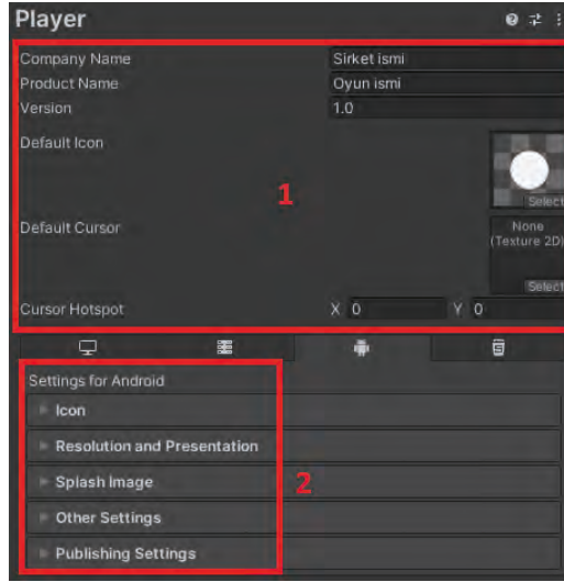
G rsel 4.59: Uygulama ayarları
