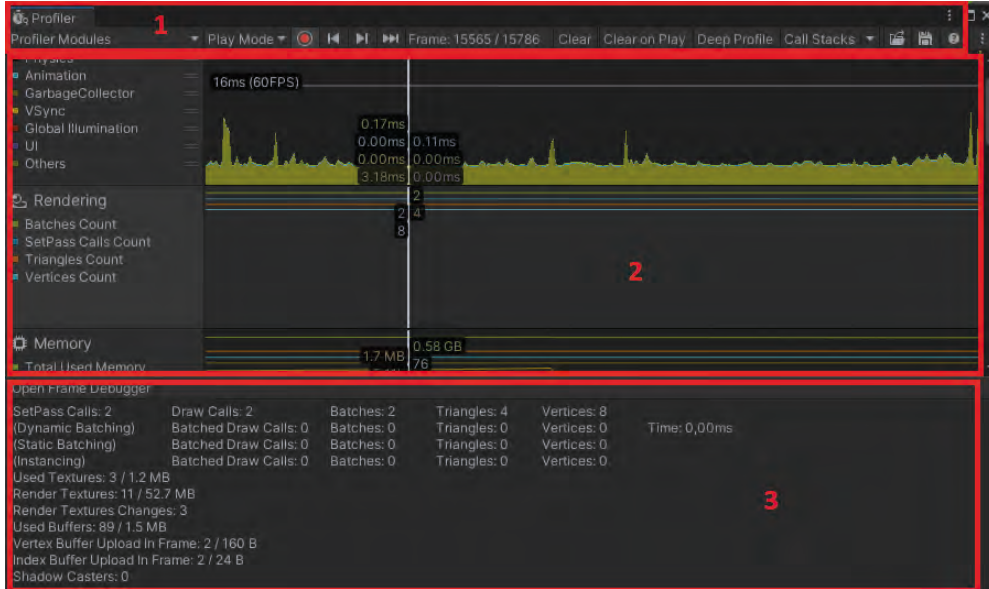
Görsel 4.52: Profiler aracı
