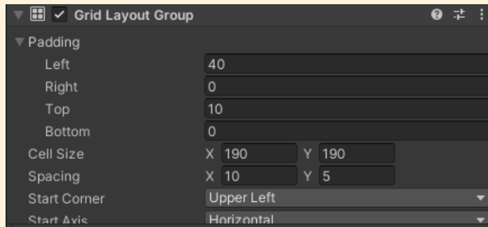
Görsel 4.26: Grid Layout Group ayarı
