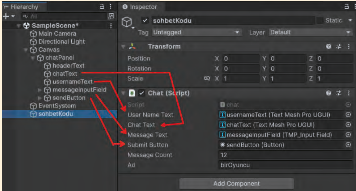
Görsel 3.126: Kod içindeki boşluklara nesnelerin atanması
