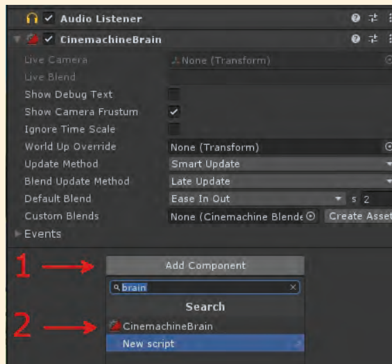
Görsel 3.5: CinemachineBrain bileşeninin eklenmesi
