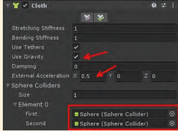
Görsel 3.52: Cloth bileşeninin ayarları
