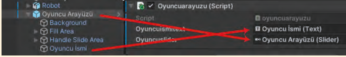
Görsel 4.18: Oyuncuarayuzu scriptindeki değişkenleri ayarlama
