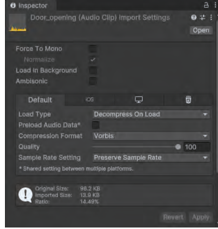
Görsel 3.148: Ses dosyasının özellikleri
