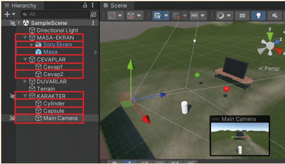
Görsel 1.80: Oyun nesnelerinin konumlarının düzenlenmesi
