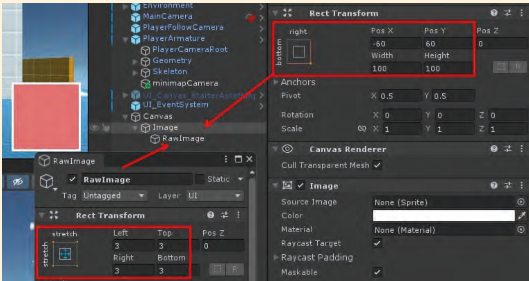
Görsel 3.99: RawImage ve Image nesnelerinin konum değerleri düzenlenir.
