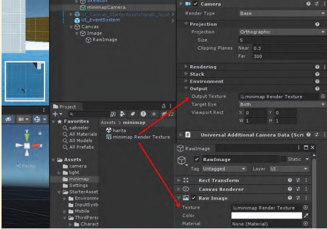
Görsel 3.100: minimapCamera’nın dokusunun düzenlenmesi
