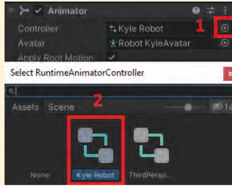
Görsel 4.14: Animator Controller özelliğinin ayarlanması
