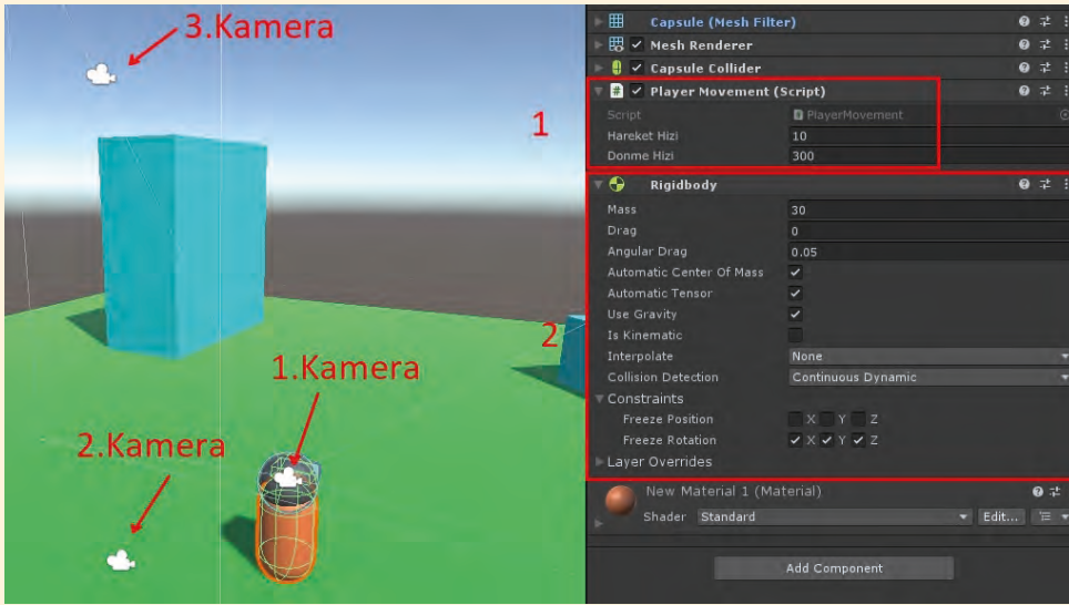
Görsel 3.94: Kod eklenir ve Rigidbody bileşeni düzenlenir.
