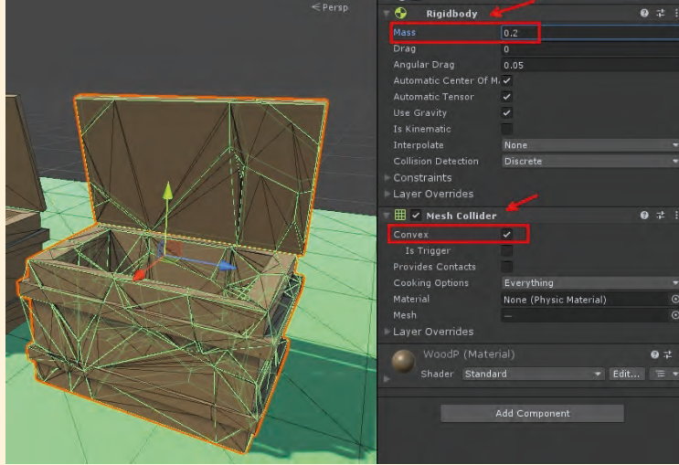
Görsel 3.57: Kırık parçalara fizik desteği ekleme
