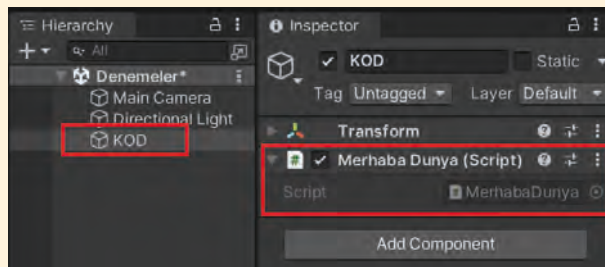
Görsel 1.73: Nesneye script dosyasının eklenmesi
