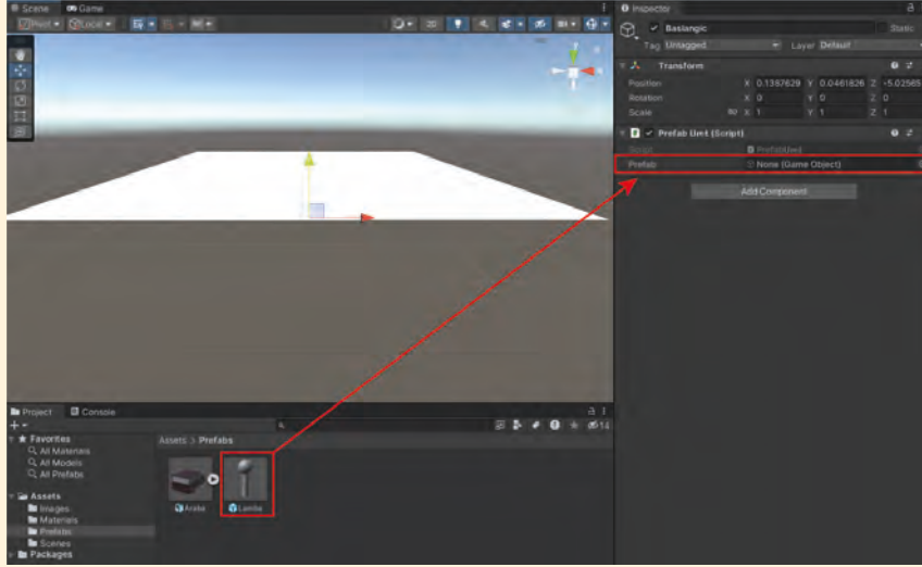
Görsel 2.86: Prefab yapısını Prefab Uret bileşeni ile ilişkilendirme
