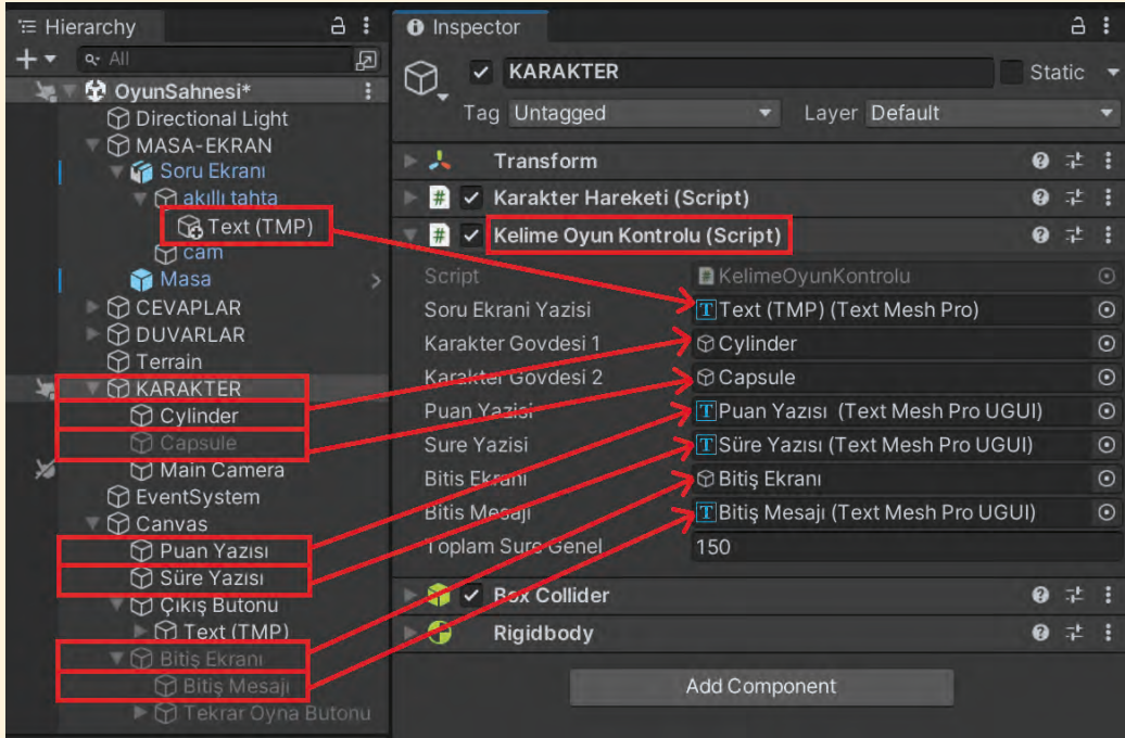
Görsel 1.117: Değişkenlere nesnelerin atanması
