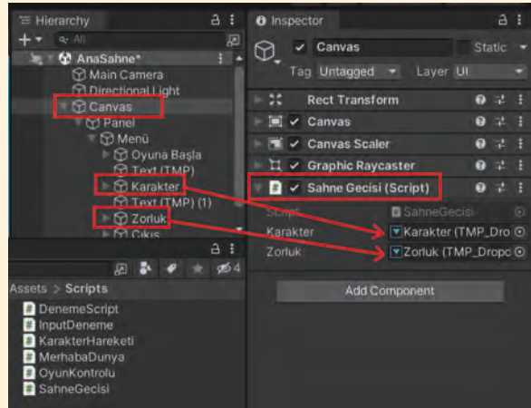
Görsel 1.104: Canvas nesnesine SahneGecisi script dosyasının eklenmesi
