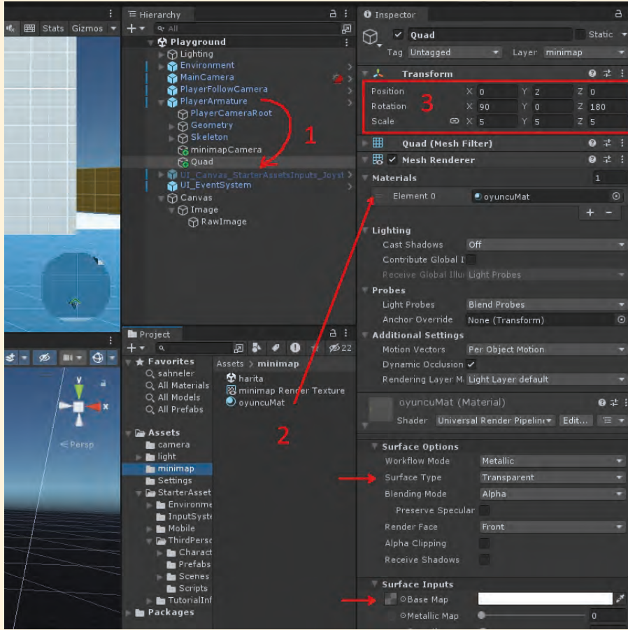
Görsel 3.102: Oyuncu içindeki Quad nesnesine yeni bir materyal oluşturma
