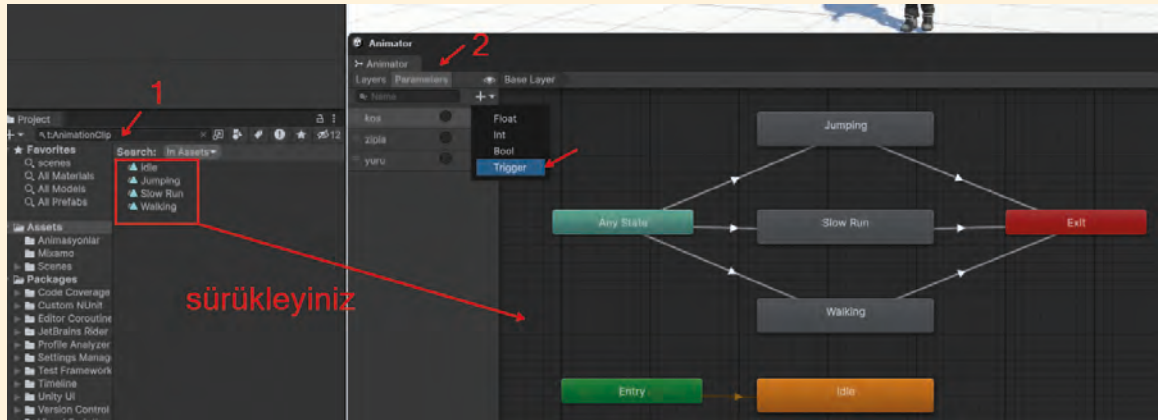
Görsel 3.39: Animasyon kliplerini Animator penceresine atıp üç adet Trigger eklenir.
