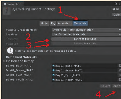
Görsel 3.31: Klasör içine doku ve materyallerin çıkarılması
