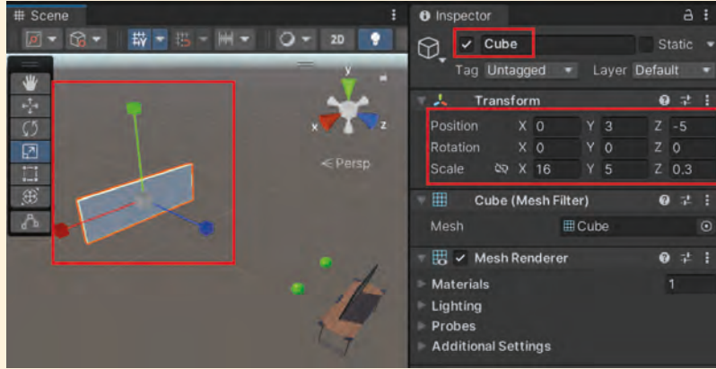
Görsel 1.49: Cube'un dönüşüm değerlerinin ayarlanması
