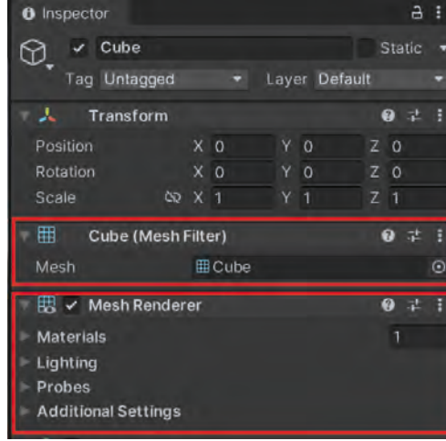
Görsel 1.23: Mesh Filter ve Mesh Renderer bileşeni
