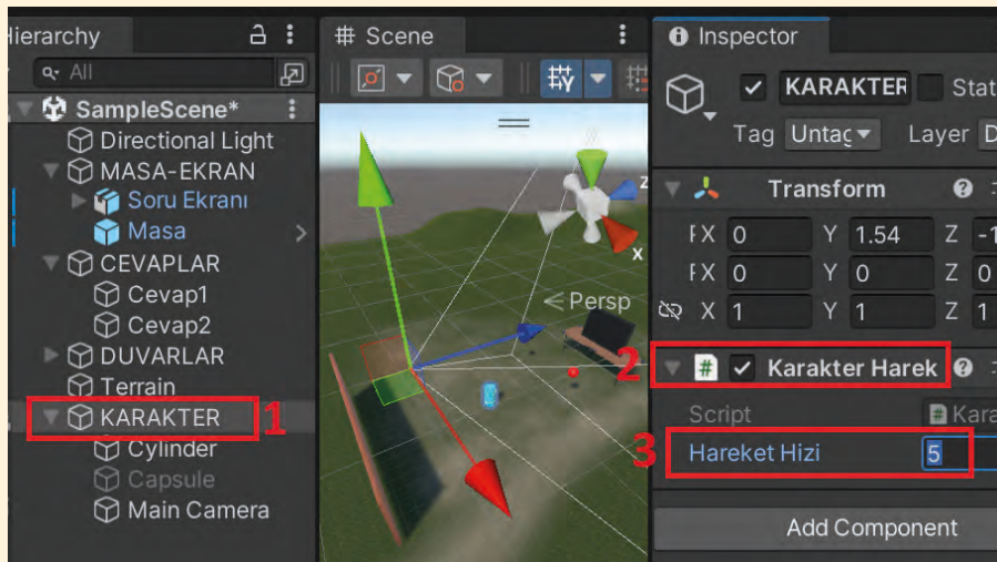
Görsel 1.82: Script dosyasının oyun nesnesine eklenmesi
