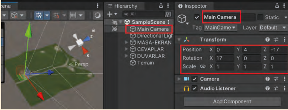
Görsel 1.67: Main Camera'nın dönüşümlerinin değiştirilmesi
