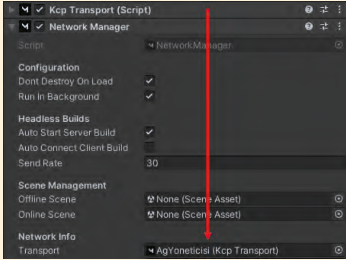
Görsel 4.7: Transport özelliğini ayarlama
