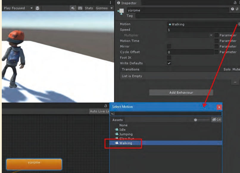
Görsel 3.38: Eklenen boş durumun adı yürüme olarak değiştirilir ve hareket (Motion) seçilir.
