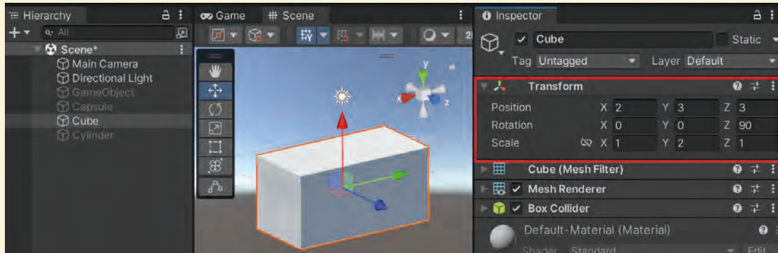
Görsel 1.18: Küpün Transform değerlerinin değiştirilmesi
