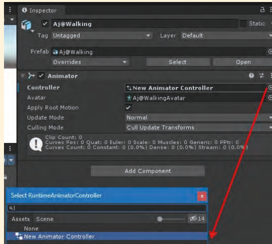
Görsel 3.36: Yeni oluşturulan kontrolcü seçilir.
