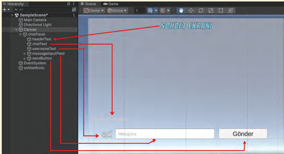
Görsel 3.125: Oyun sahnesindeki gerekli nesneler
