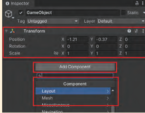
Görsel 1.8: Oyun nesnesine ait Inspector paneli
