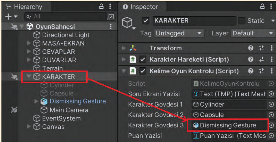
Görsel 2.79: Hazır karakter modelinin referans değişkene atanması
