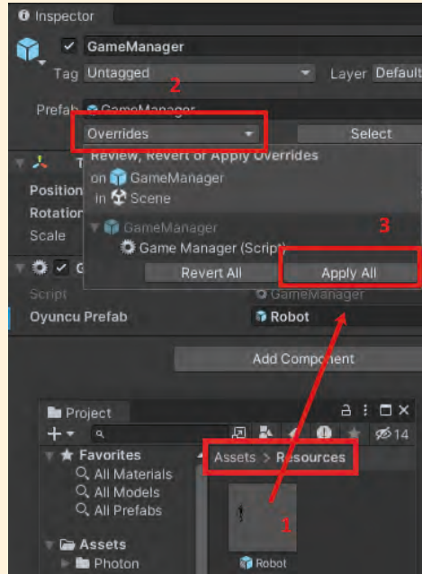
Görsel 4.20: GameManager bileşenini ekleme
