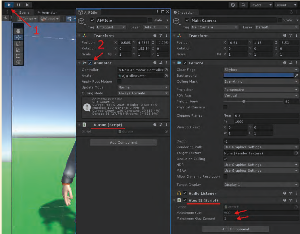
Görsel 3.78: Ragdoll etkisi için kodları ekleme
