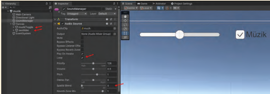
Görsel 3.152: Slider ve Toggle nesneleri eklenir.
