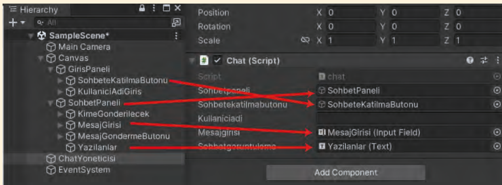
Görsel 4.50: ChatYoneticisi nesnesinin değişkenlerini ayarlama
