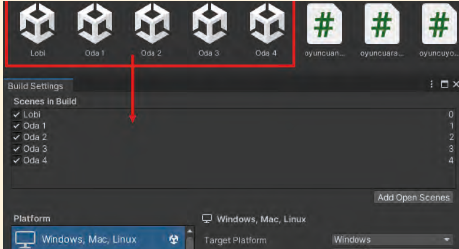
Görsel 4.21: Sahnelerin derlemeye dâhil edilmesi
