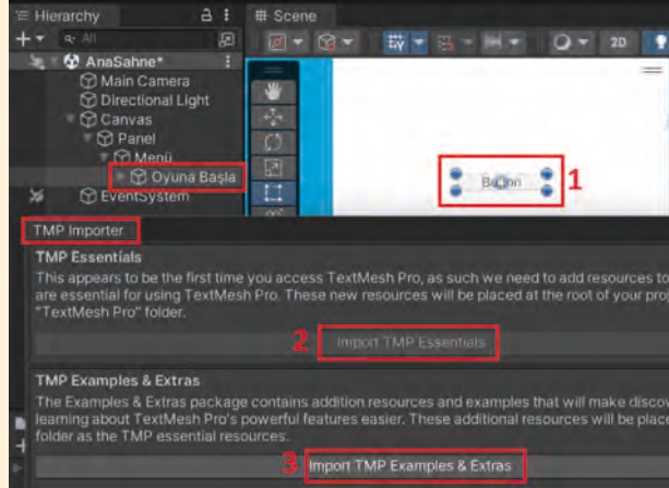
Görsel 1.95: Butonun eklemesi ve TextMeshPro'nun yüklenmesi
