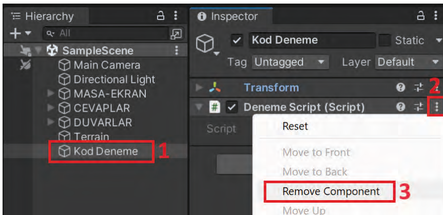
Görsel 1.70: Oyun nesnesinden bileşenin kaldırılması
