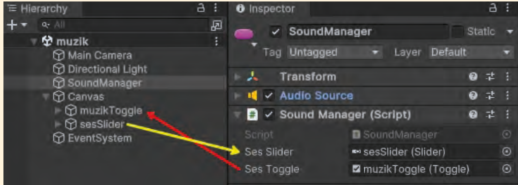
Görsel 3.153: Gerekli nesnelerin bağlanması
