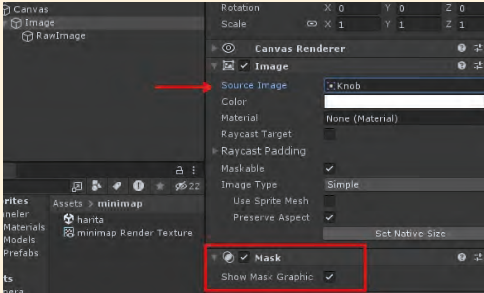
Görsel 3.101: Mask bileşeni eklenir ve Source Image seçilir.
