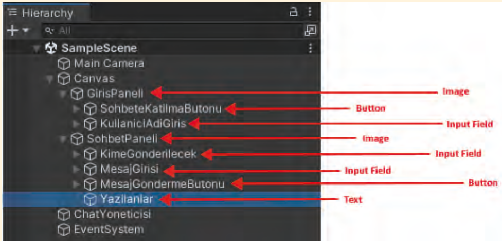
Görsel 4.48: Arayüz hazırlama
