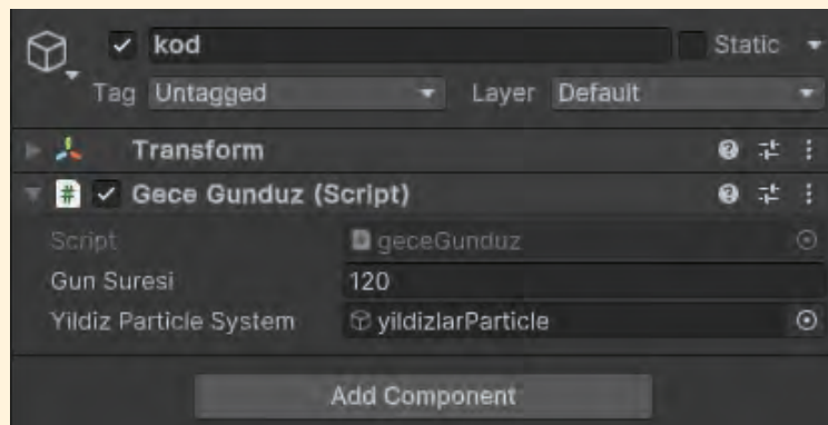
Görsel 3.132: Gece gündüz kodundaki özellikler
