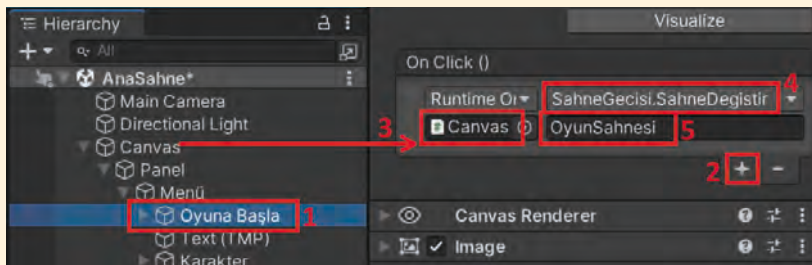
Görsel 1.105: Oyuna Başla butonun tıklama olayının ayarlanması
