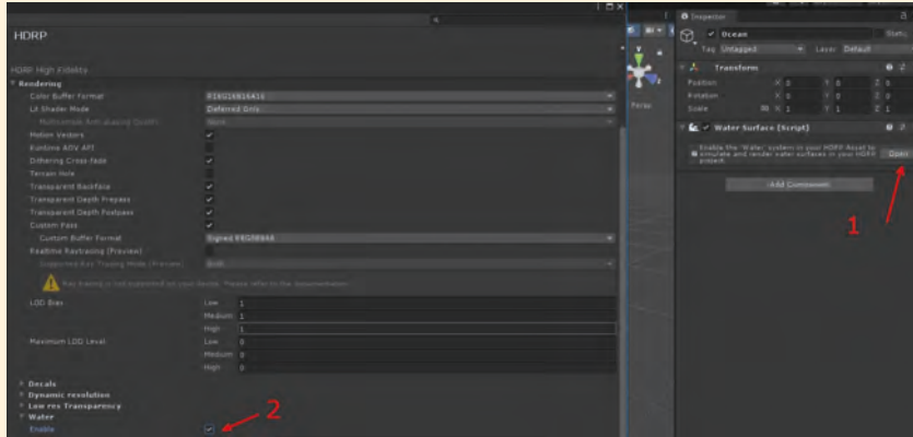
Görsel 3.63: Su yüzeyinin görüntülenmesi için gereken ayar yapılır.
