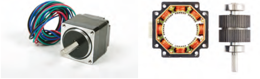
Görsel 3.59: Step Motor dış ve iç görünüşü
