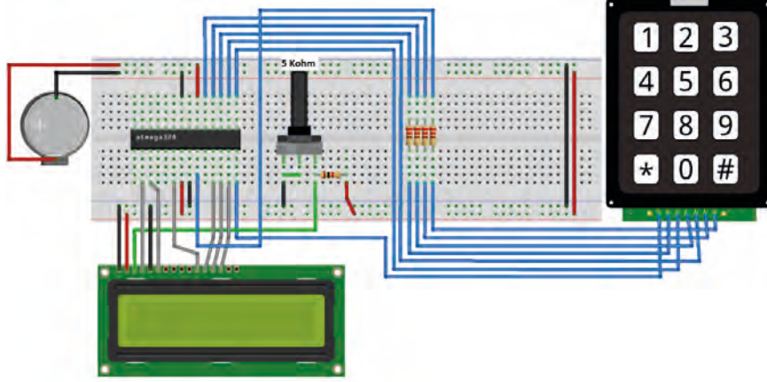
Görsel 3.31: 3.7 No.lu uygulama için breadboard eleman dizilimi
