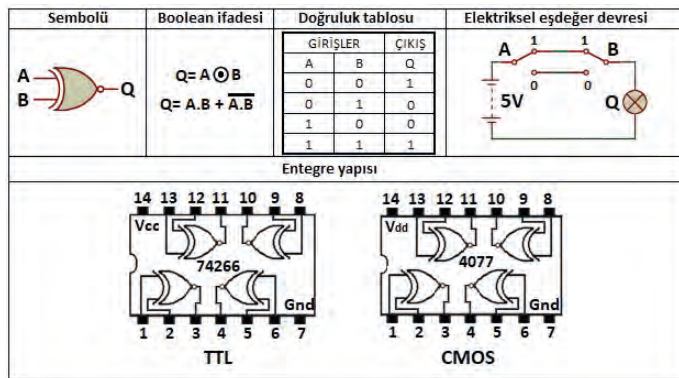
Görsel 1.21: ÖZEL VEYA DEĞİL kapısı
