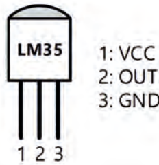
Görsel 4.72: LM35 bacak bağlantısı
