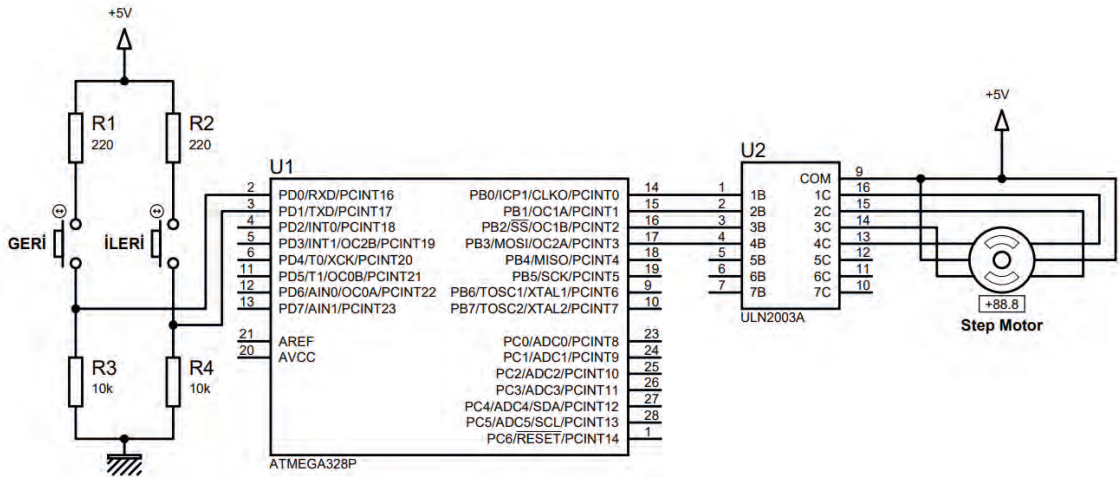
Görsel 3.60: 3.13 No.lu uygulama için simülasyon devre şeması
