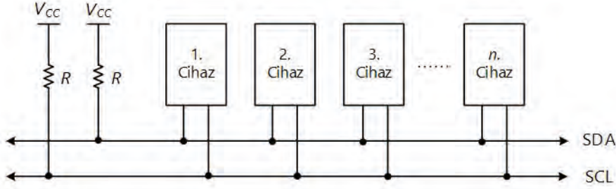
Görsel 3.82: TWI aygıtlar arası bağlantısı
