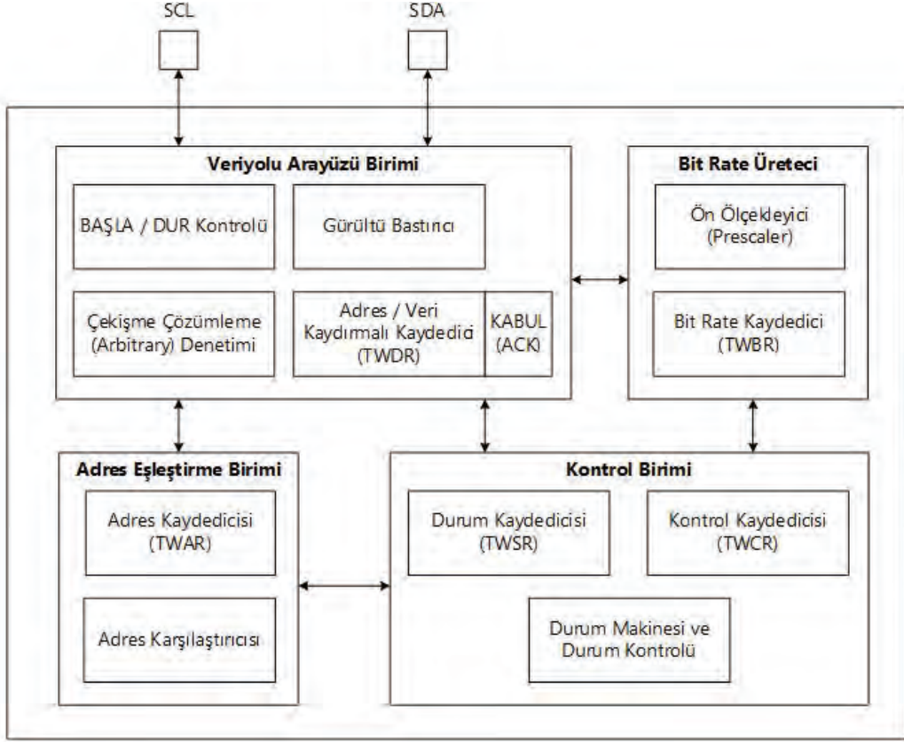
Görsel 3.87: TWI modülü blok şeması
