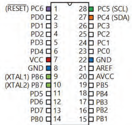
Görsel 3.88: Atmega328P mikrodenetleyicinin TWI modülü ile ilgili pinleri
