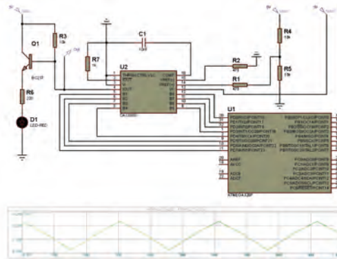
Görsel 4.30: Uygulama 4.4 için simülasyon devresi
