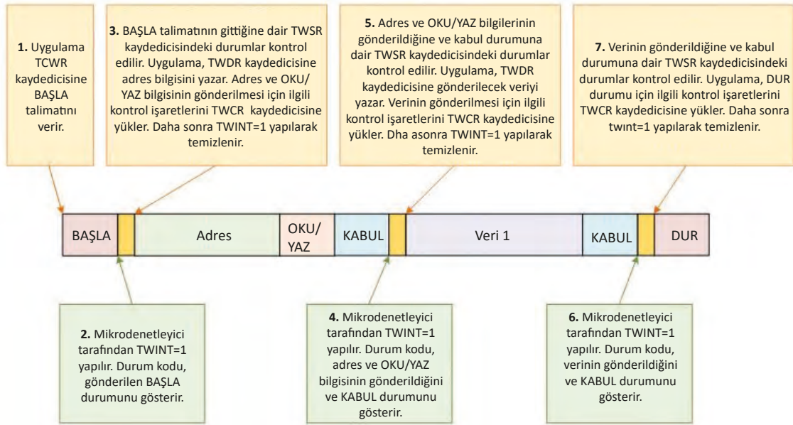
Görsel 3.95: TWI master gönderici modu veri aktarımı işlem adımları
