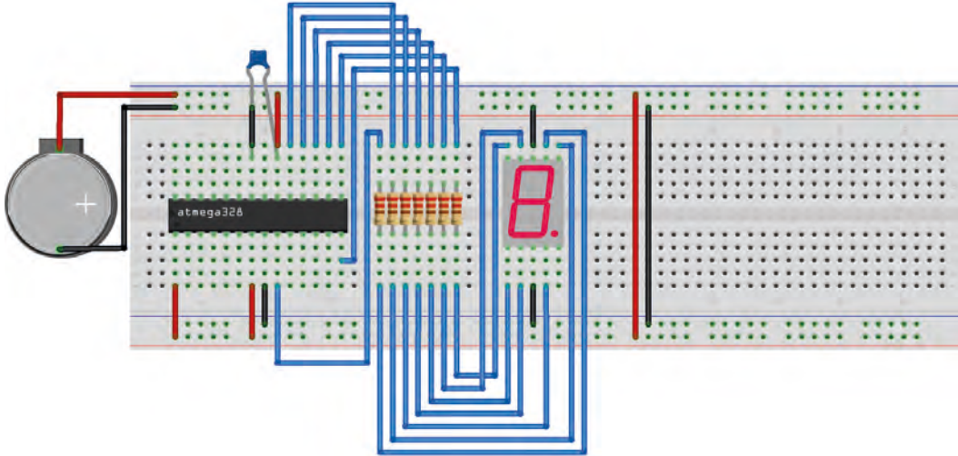
Görsel 3.8: 3.2 No.lu uygulama için breadboard eleman dizilimi
