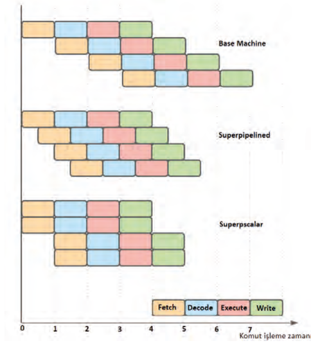
Görsel 2.18: Komut işleme aşamaları
