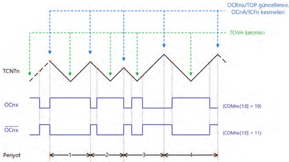
Görsel 4.49: Doğru faz PWM modu zamanlama diyagramı
