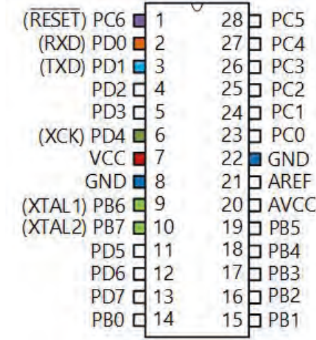
Görsel 3.72: Atmega328P mikrodenetleyicinin USART modülü ile ilgili pinleri
