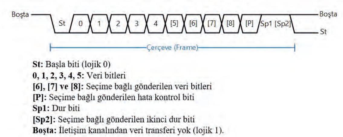
Görsel 3.74: USART çerçeve formatı
