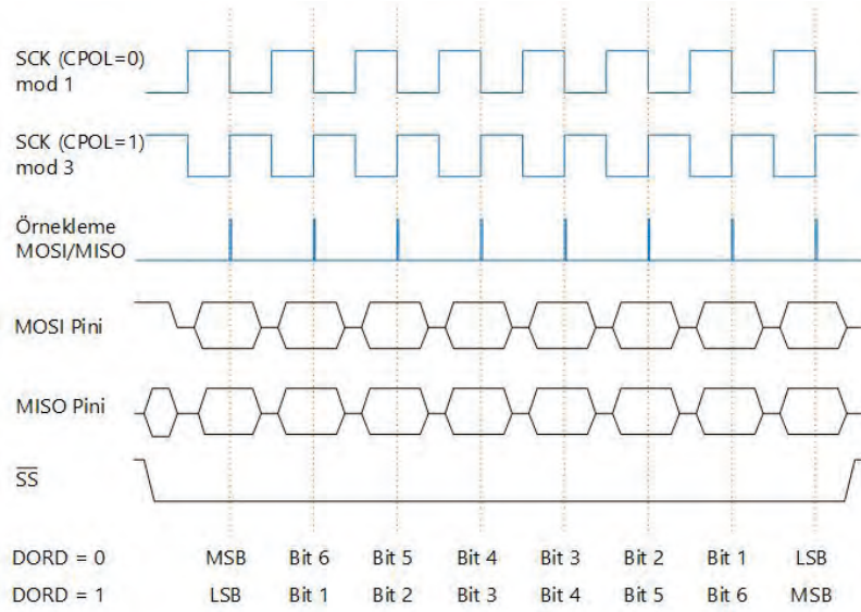
Görsel 3.66: CPHA = 1 iken SPI veri aktarım formatı
