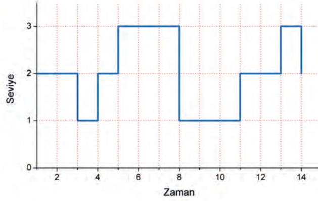
Görsel 4.4: Kuantalama yapılan işaret
