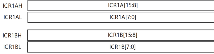
Görsel 4.56: ICR1A ve ICR1B Giriş yakalama kaydedicileri
