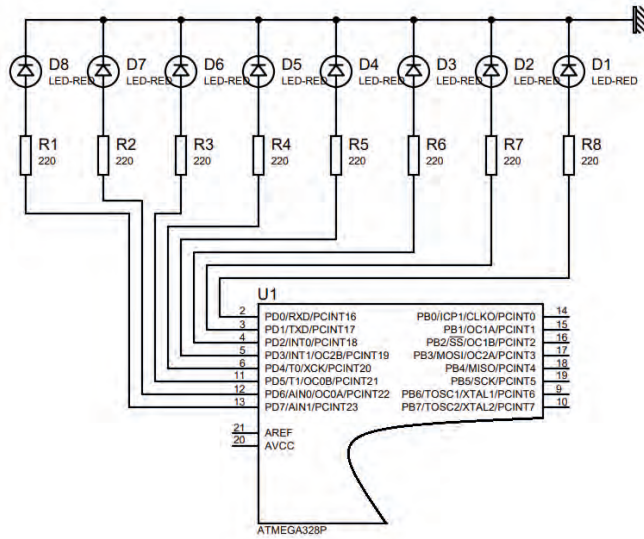
Görsel 2.73: 2.4 No.lu uygulama için simülasyon devre şeması
