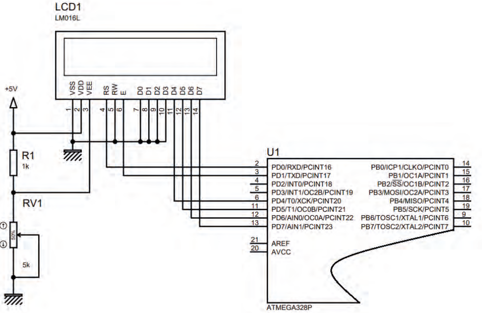
Görsel 3.29: Uygulama devresi
