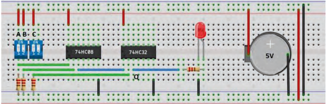
Görsel 1.40: Q = AB + C lojik ifadesinin devresi
