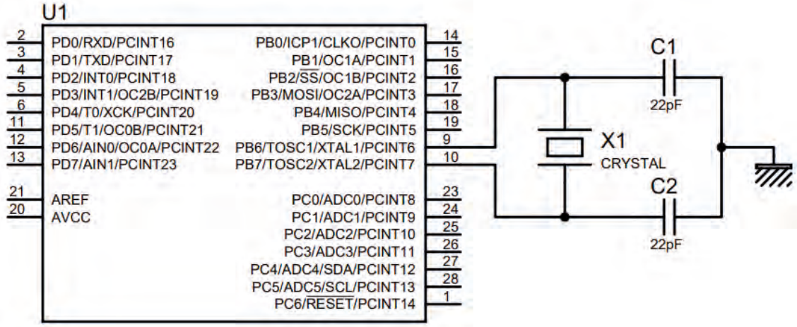
Görsel 2.21: Mikrodenetleyiciye kristal osilatör bağlama
