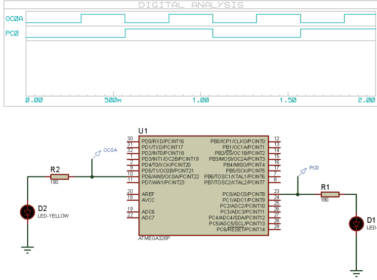
Görsel 4.43: Uygulama 4.5 için simülasyon devre şeması
