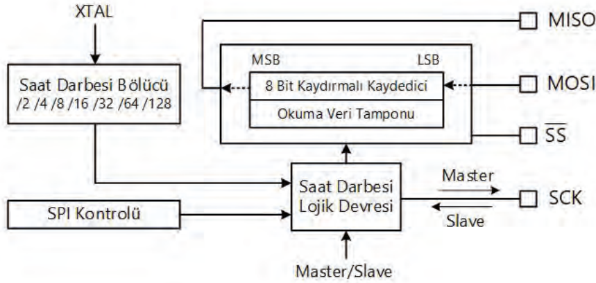
Görsel 3.62: SPI haberleşme modülü basitleştirilmiş blok şeması
