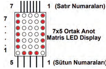
Görsel 3.16: Matris Display LED (U harfi)
