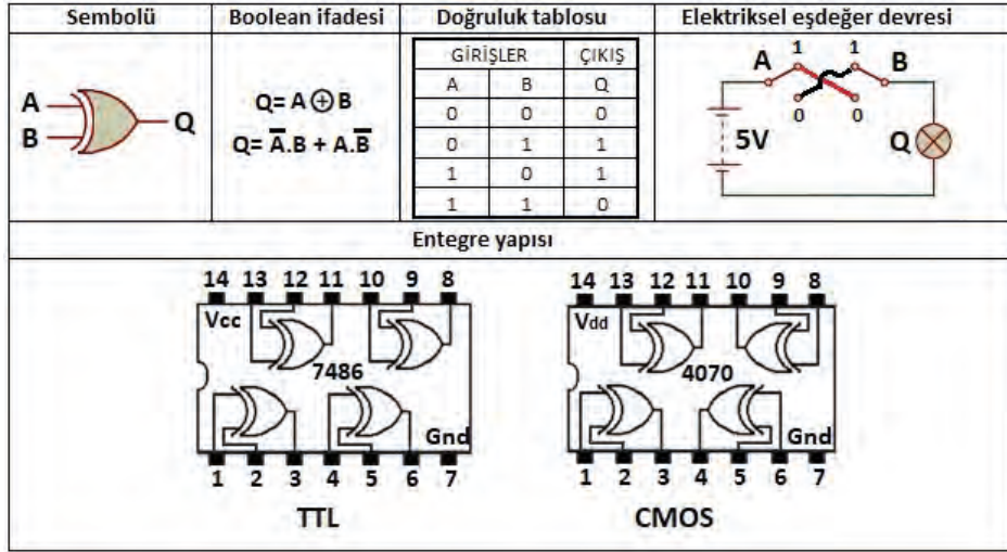
Görsel 1.19: ÖZEL VEYA kapısı
