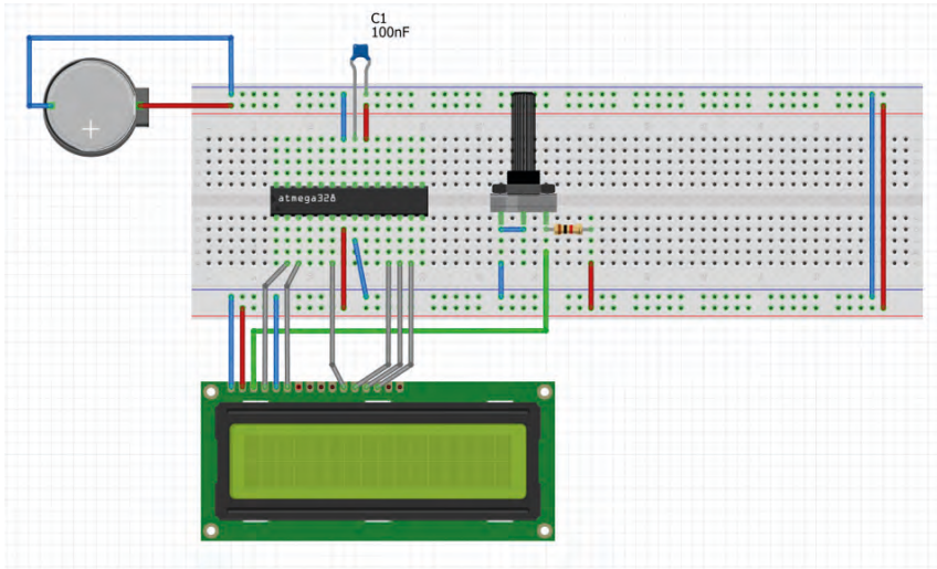
Görsel 4.69: Uygulama 4.10 için breadboard üzerindeki devre
