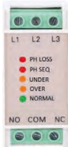
Görsel 3.40: Faz koruma rölesi
