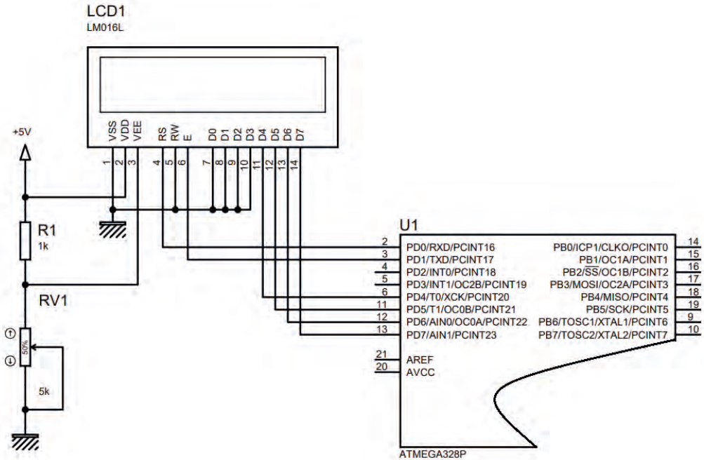
Görsel 3.27: 3.7 No.lu uygulama için simülasyon devre şeması
