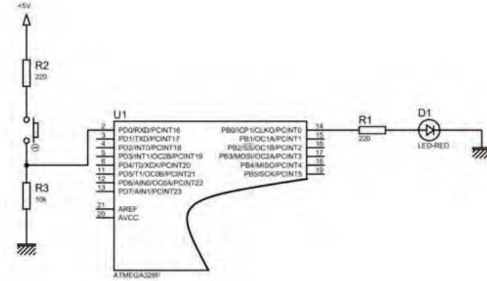
Görsel 2.72: Uygulama devresi
