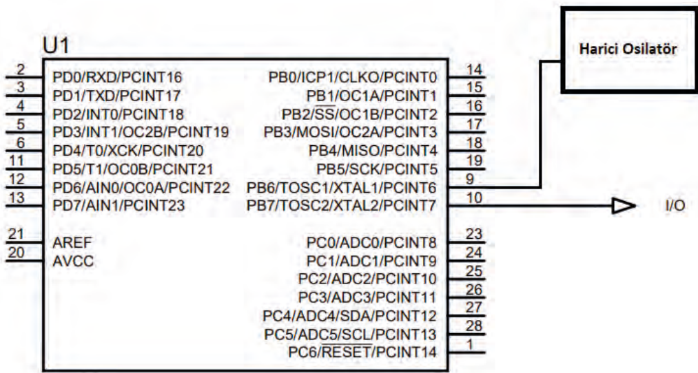
Görsel 2.24: EC osilatör bağlantısı
