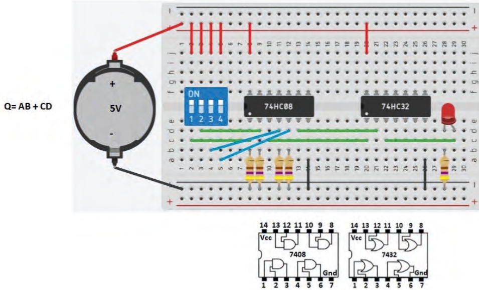
Görsel 1.43: Breadboard üzerine lojik devre kurulması
