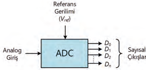
Görsel 4.6: ADC blok şeması
