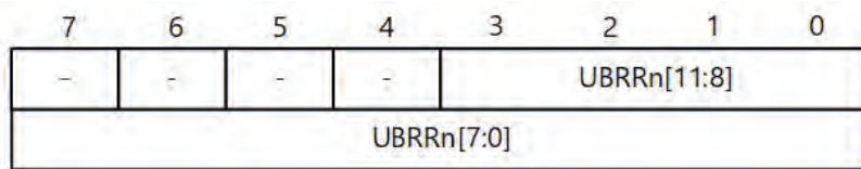
Görsel 3.79: UBRRn kaydedicisi
