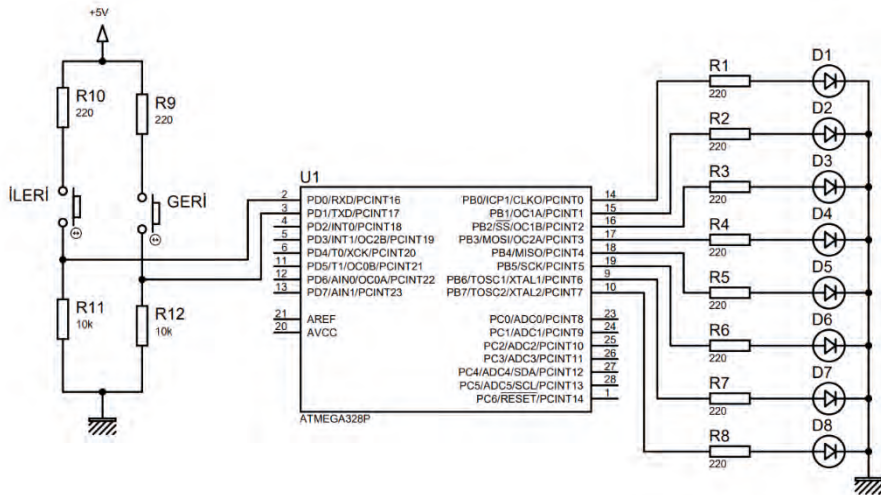
Görsel 2.78: 2.6 No.lu uygulama için simülasyon devre şeması
