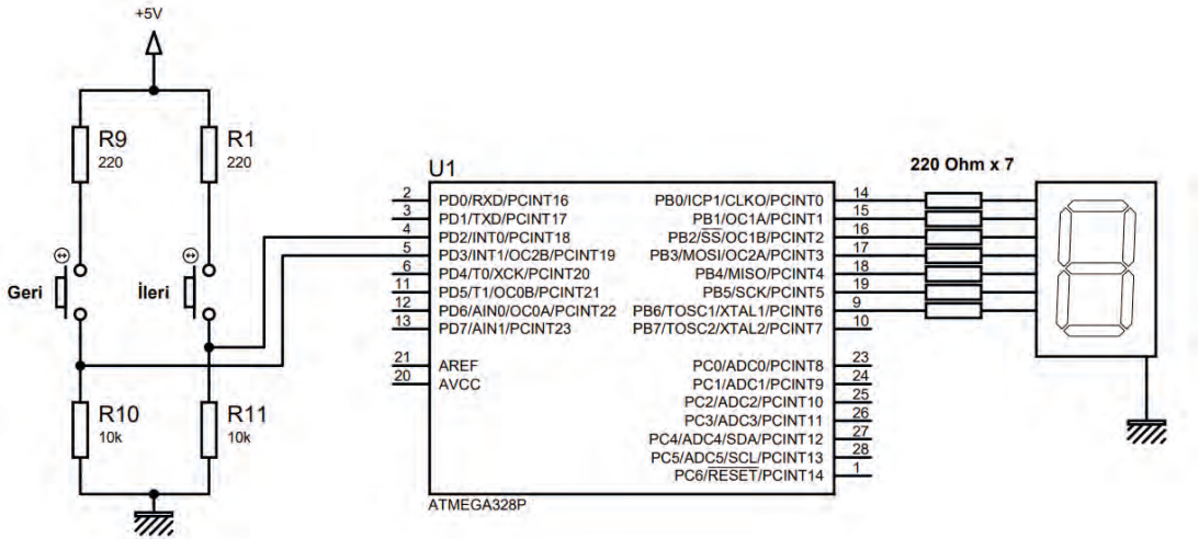
Görsel 3.10: 3.3 No.lu uygulama için simülasyon devre şeması
