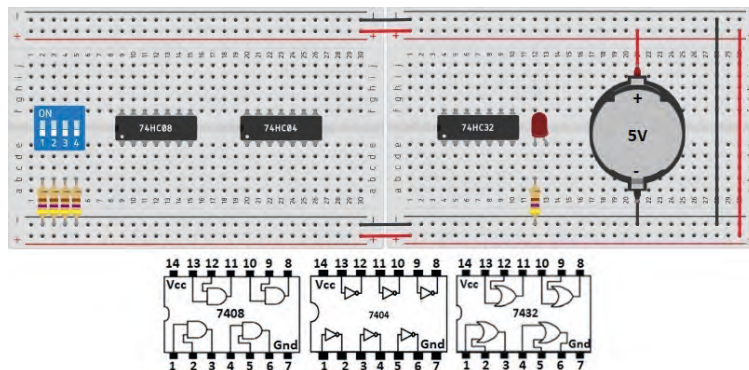
Görsel 1.57: Breadboard üzerine kurulacak uygulama devresi
