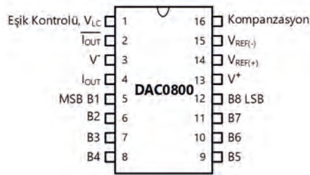
Görsel 4.28: DAC0800 entegresi DIP soket pin şeması
