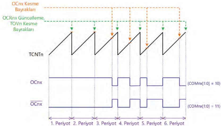
Görsel 4.36: Hızlı PWM modu zamanlama diyagramı
