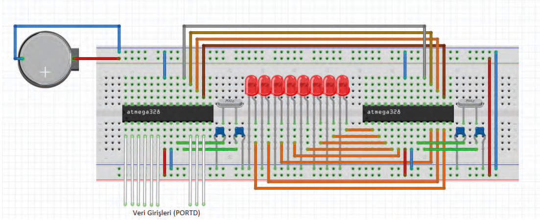
Görsel 3.70: 3.14 No.lu uygulama için breadboard üzerine kurulan devre
