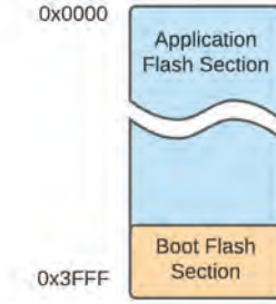
Görsel 2.8: Atmega328P Program belleği haritası
