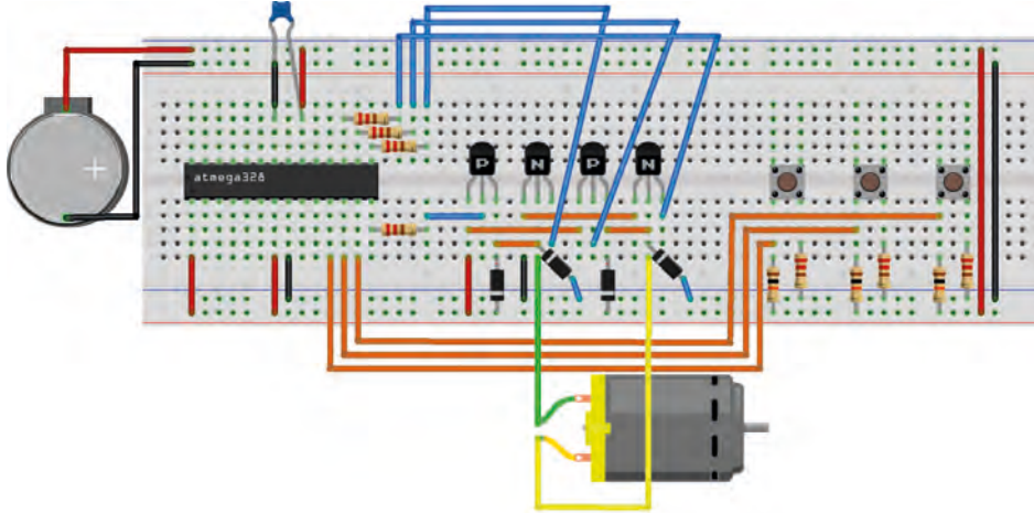
GörSEL 3.55: 3.11 No.lu uygulama için breadboard eleman dizilimi
