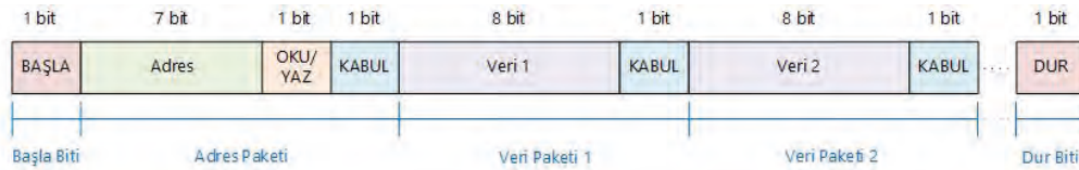
Görsel 3.86: Adres ve veri aktarım formatı
