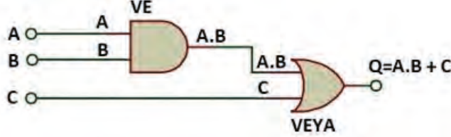
Görsel 1.39: Q = AB + C lojik ifadesinin şeması
