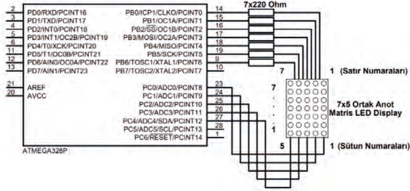
Görsel 3.22: Uygulama devresi
