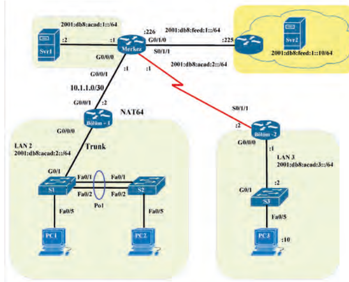
Görsel 2. 11: Mantıksal IPv4 ve IPV6 ağ topolojisi
