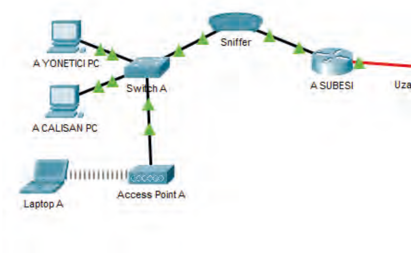
Görsel 3.28 Sniffer cihazı bağlantısı
