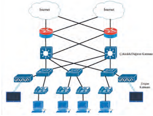
Görsel 2. 1: İki katmanlı model
