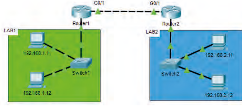
Görsel 3.5: Yönlendirme
