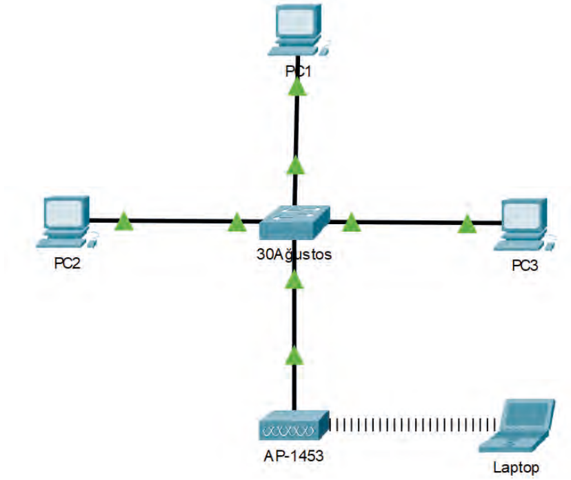
Görsel 3.16: Kablosuz ağ simülasyonu
