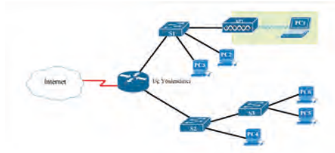
Görsel 2. 4: Hata etki alanı
