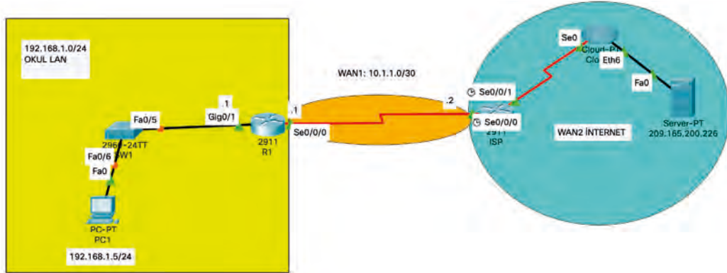
Görsel 2.15: Ağ topolojisi
