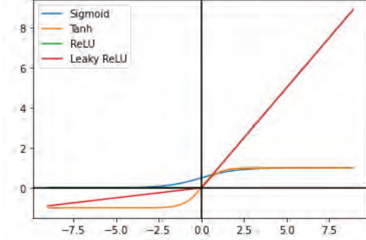
Görsel 3.15: Aktivasyon fonksiyonları grafikleri
