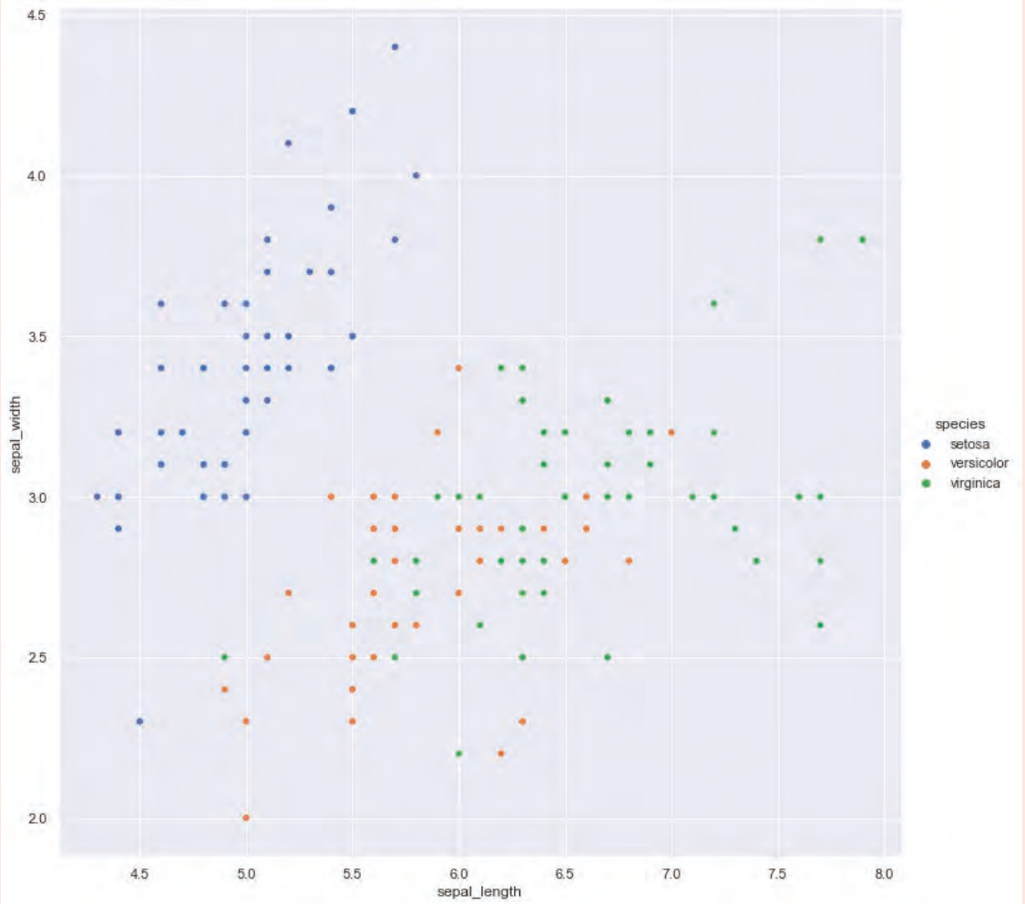
Görsel 2.32: İris veri seti türlerine göre çanak yaprağı saçılım grafiği
