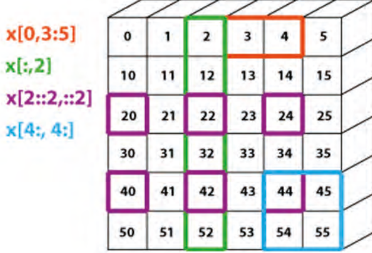
Görsel 1.30: NumPy dilimleme ve indeksleme
