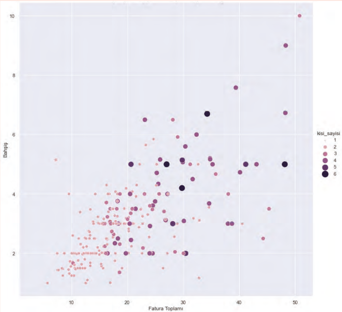
Görsel 2.23: Kişi sayısı bahşiş–fatura toplamı saçılım grafiği
