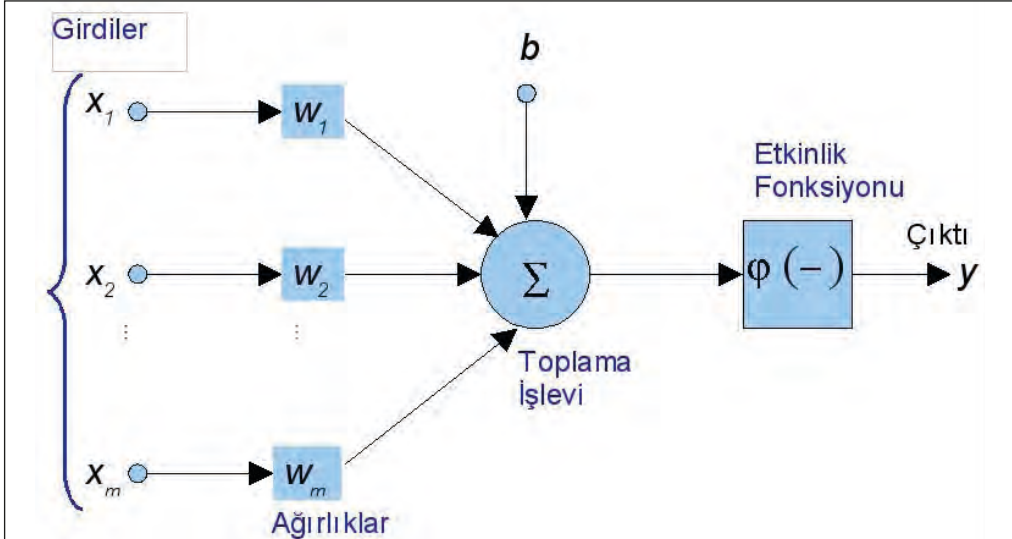
Görsel 3.5: Bir sinir hücresinin matematiksel modeli
