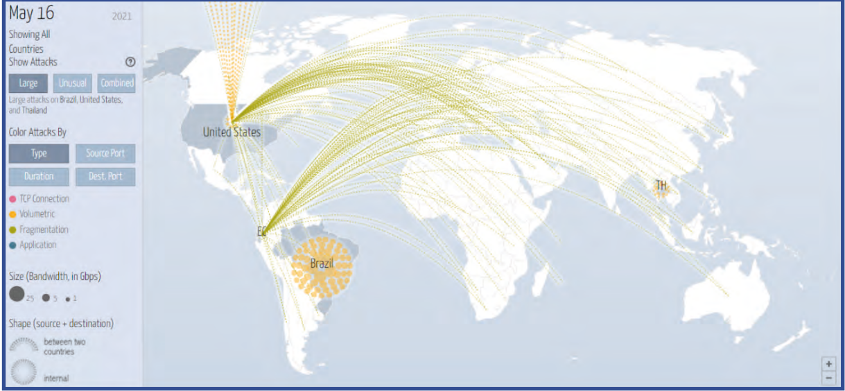
Görsel 8.9: DDoS saldırı haritası
