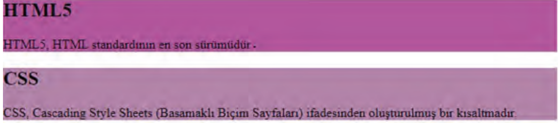
Görsel 3.28: <section> etiketi kullanımı
